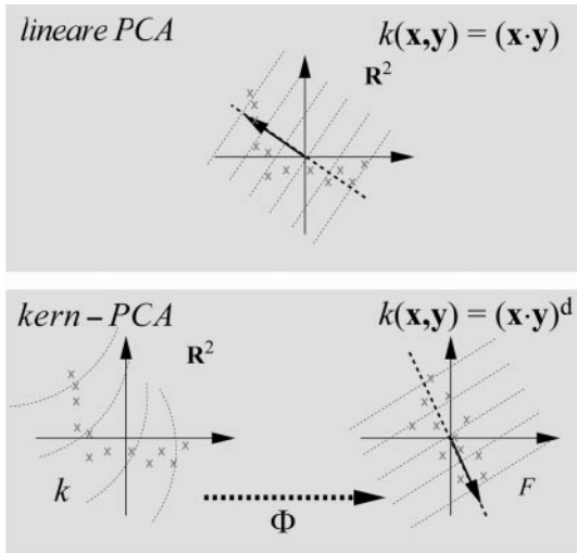
Abb. 4. Durch Verwendung einer Kernfunktion führt Kern-PCA implizit eine lineare PCA in einem hochdimensionalen Raum durch, der nichtlinear mit dem Ursprungsraum zusammenhängt [27]
