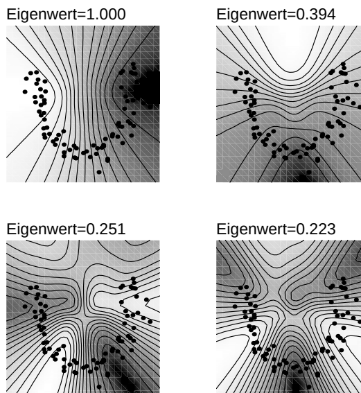
Abb. 6. Darstellung der ersten 4 nichtlinearen Merkmalsextraktoren bei Kern-PCA mit Sigmoid-Kern (17) auf dem Datensatz aus Abb. 5. Die Komponenten extrahieren nichtlineare Struktur aus dem Datensatz; so passt sich beispielsweise der erste Extraktor (links oben) besser der Krümmung der Daten an als die entsprechende Komponente in Abb. 5
