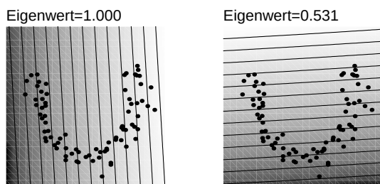
Abb. 5. Lineare PCA, oder, äquivalent, Kern-PCA mit k(\mathbf{x}, \mathbf{y}) = (\mathbf{x} \cdot \mathbf{y}) . Darstellung der zwei linearen Merkmalsextraktoren auf einem künstlichen Datensatz (entsprechend den beiden Eigenvektoren, nach Größe der Eigenwerte sortiert). Spezifische Grauwerte und Höhenlinien kennzeichnen Gebiete, wo (29) gleiche Werte annimmt. Der erste Extraktor (links) projiziert auf die Richtung maximaler Varianz in den Daten, und verdeutlicht, dass man allein durch Betrachtung der Varianz im Eingaberaum bei dem zugrundeliegenden Datensatz die nichtlineare Struktur nicht angemessen identifizieren kann
