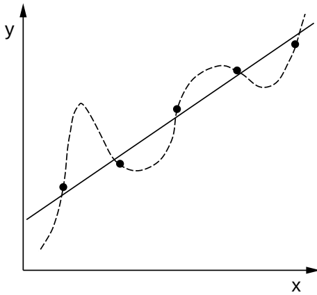
Abb. 1. Aus einer gegebenen Menge von Beispielen (im Bild: schwarze Punkte) soll ein unbekannter funktionaler Zusammenhang geschätzt werden. Die statistische Lerntheorie formalisiert, in welchem Sinne die Gerade als Schätzung vorzuziehen ist (siehe Text)
