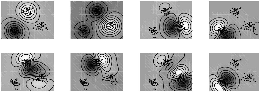
Abb. 7. Darstellung der ersten 8 nichtlinearen Merkmalsextraktoren, die man durch Anwendung von Kern-PCA mit RBF-Kern (18) auf einen künstlichen Datensatz aus drei Gauß-Clustern erhält (aus [27]). Links oben: die ersten beiden Komponenten teilen die Daten in drei Cluster auf. (Dies geschieht, obwohl der Algorithmus nicht explizit die Clusterung zum Ziel hat.) Diese nichtlineare Struktur in den Daten trägt dementsprechend im Merkmalsraum maximale Varianz. Die höheren Komponenten untersuchen die verbleibende Varianz, die darin besteht, dass die Cluster ausgedehnt sind. Komponenten 3–5 halbieren jeweils einen Cluster, wie auch 6–8, letztere orthogonal zu den vorherigen Halbierungen
