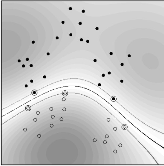
Abb. 3. Beispiel eines SV-Klassifikators mit RBF-Kern (18). Kreise und Punkte stellen zwei Klassen von Trainingsbeispielen dar. Die mittlere Linie ist die Entscheidungsgrenze, die äußeren Linien kennzeichnen diejenigen Beispiele, die in F am dichtesten an der separierenden Hyperebene liegen. Die Support-Vektoren, die der Algorithmus findet (eingekreist), sind nicht Clusterzentren, sondern Beispiele, die für die Lösung der gegebenen Klassifikationsaufgabe kritisch sind
